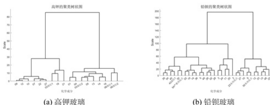
图 2 Q 型聚类结果
