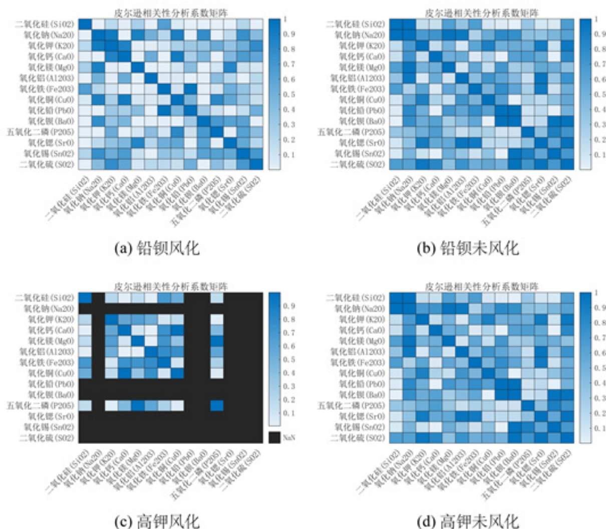
图 6 四类相关系数矩阵
